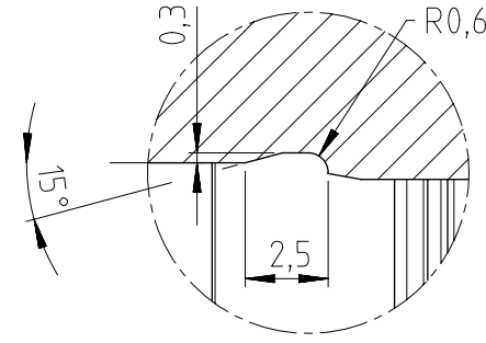
DETAY C ÖLÇEK 4:1
