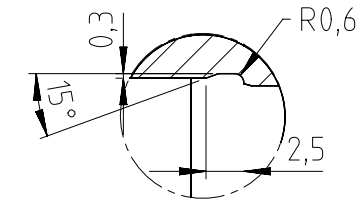
DETAY B ÖLÇEK 2:1
