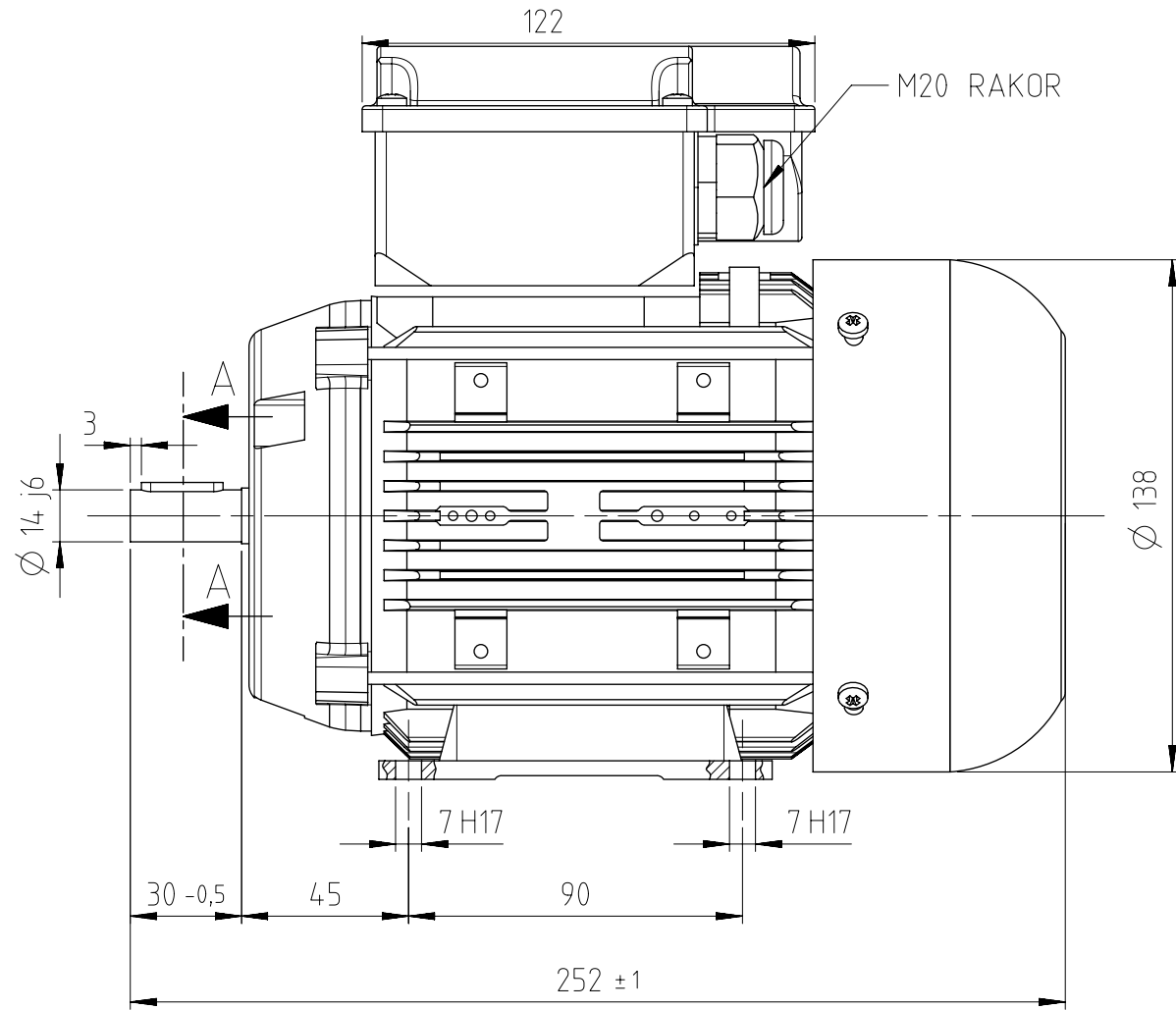
KESİT A-A ÖLÇEK 1:1
