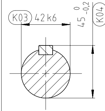
KESİT A-A ÖLÇEK 1:2
