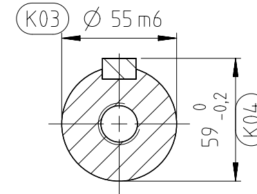
KESİT A-A ÖLÇEK 2:5
