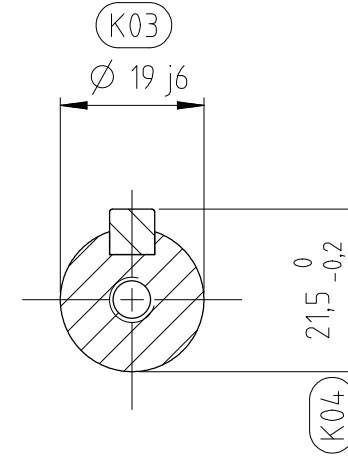
KESİT A-A ÖLÇEK 1:1
