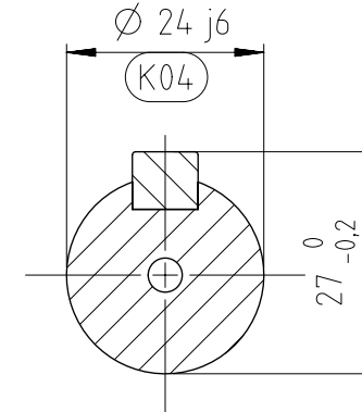
KESİT A-A ÖLÇEK 1:1
