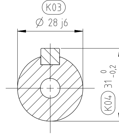
KESİT A-A ÖLÇEK 1:1
