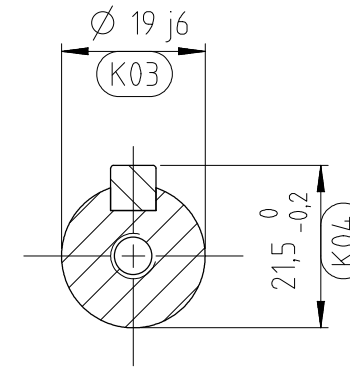
KESİT A-A ÖLÇEK 1:1
