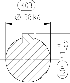
KESİT A-A ÖLÇEK 2:3
