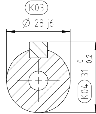
KESİT A-A ÖLÇEK 1:1
