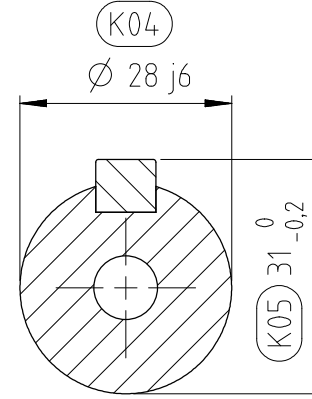
KESİT A-A ÖLÇEK 1:1
