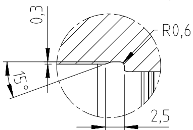
DETAY B ÖLÇEK 2:1
