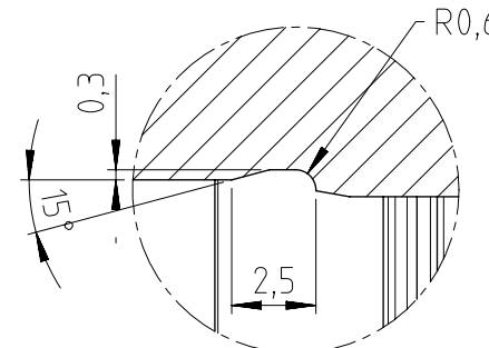
DETAY C ÖLÇEK 4:1
