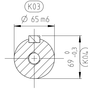
KESİT A-A ÖLÇEK 1:3
