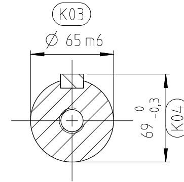
KESİT A-A ÖLÇEK 1:3
