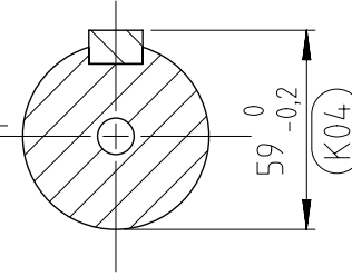
KESİT A-A ÖLÇEK 2:5
