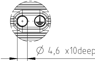
DETAY B ÖLÇEK 1:1
